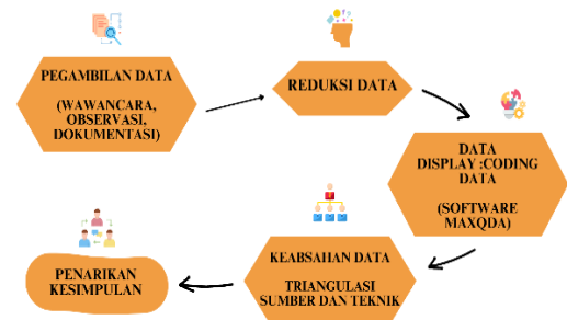
Gambar 1. Analisis Data
